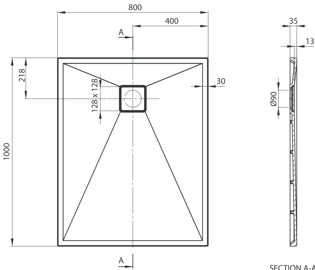
SECTION A-A
