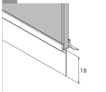
c USZCZELKA PROGOWA
