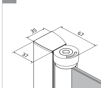
a PROFIL PRZYŚCIENNY
