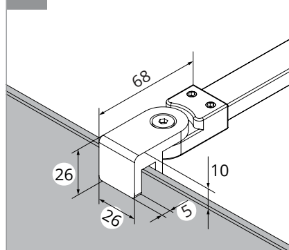
c WSPORNIK
