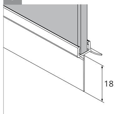
d USZCZELKA PROGOWA
