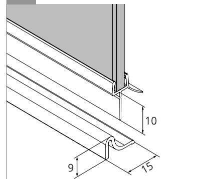
h MONTAŻ Z PROGIEM
