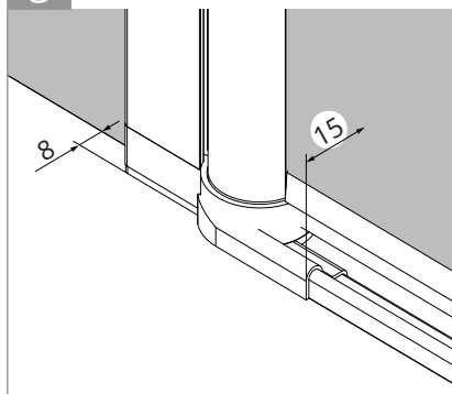
g ZAKOŃCZENIE PROGU
