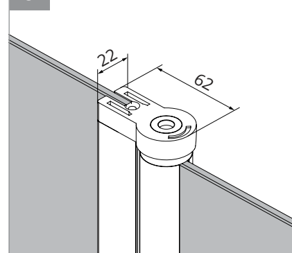
d ZAWIAS KOLUMNOWY
