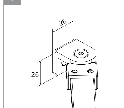
b WSPORNIK
