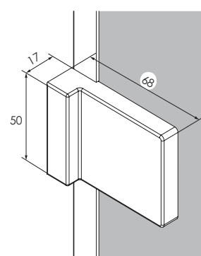
d KOSTKA MONTAŻOWA
