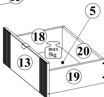
SZAFKA P./UM 2SZ 80
